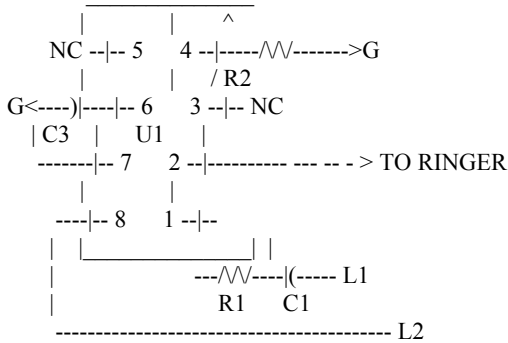
a. Main ringer TTL circuit
